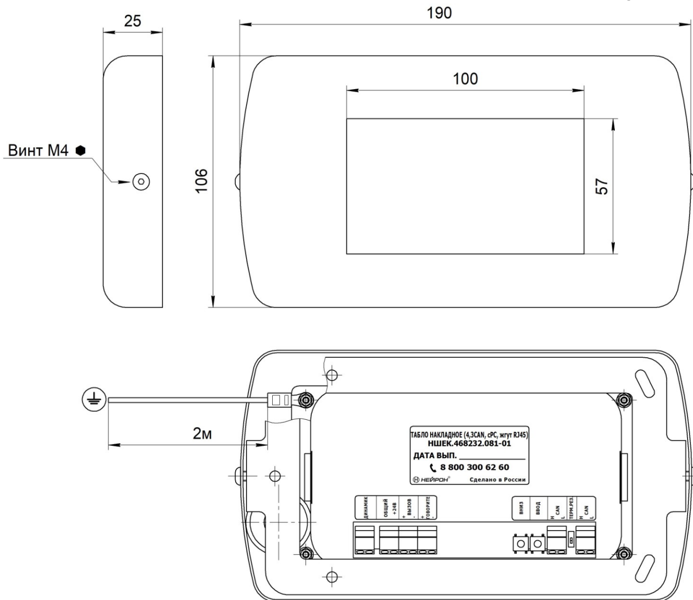
Рис.1 Внешний вид Табло накладное (4,3CAN, сРС, жгут RJ45) НШЕК.468232.081-01
